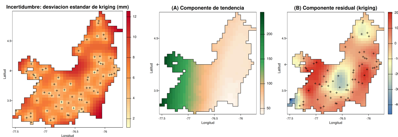
Figura 10. Izquierda: desviación estándar de kriging. Se comporta como manda la teoría — mínima sobre las estaciones (1,1 mm), creciente con la distancia al dato más cercano y máxima en los bordes y en los huecos sin muestrear (12,6 mm en el filo oriental, la punta norte y la cintura del departamento). Este mapa solo es legible porque sd(z) = 1,06 ; con el modelo de menor RMSE habría exagerado la precisión. Derecha: la respuesta gráfica al enunciado. (A) es lo que aporta la tendencia determinística y (B) lo que agrega el kriging del residuo. El panel B no es ruido : tiene estructura espacial organizada, y esa estructura es precisamente "el papel de la correlación espacial" que había que evaluar.
