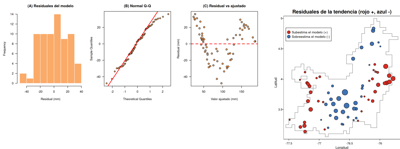
Figura 5. Izquierda: diagnóstico de los residuales. El Q-Q sigue la recta con colas ligeramente cortas, pero el panel de residuales contra ajustados dibuja una U clara (ajustado \approx 30 \rightarrow residual +30 ; ajustado \approx 100 \rightarrow residual -40 ; ajustado \approx 170 \rightarrow residual +25 ). Es curvatura sistemática: la tendencia lineal en longitud está mal especificada. Derecha: esos mismos residuales sobre el mapa. No están dispersos al azar sino agrupados en manchas — el modelo sobreestima en el centro del valle y en el norte, y subestima en los dos flancos. Es la U del panel anterior vista en el espacio: una recta no puede curvarse, así que aplana el fondo del valle hacia arriba y las laderas hacia abajo. Este mapa anticipa el resultado de la sección 4.
