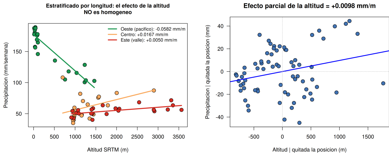
Figura 4. Izquierda: la relación altitud-precipitación estratificada por tercil de longitud. Agrupando los 70 puntos la pendiente es -0,0369 mm/m, pero dentro de cada banda cambia: oeste -0,0582 , centro +0,0167 , este +0,0050 . En el Chocó el máximo de lluvia está al nivel del mar porque la masa húmeda es somera y descarga abajo; en las laderas interiores manda el ascenso orográfico y la lluvia sube con la altura. Derecha: gráfico de variable añadida, con los residuales de precipitación y de altitud después de quitarle a ambos la posición. Su pendiente, +0,0098 , es exactamente el coeficiente de la tabla 4, y es el efecto real de la altitud una vez descontada la longitud.
