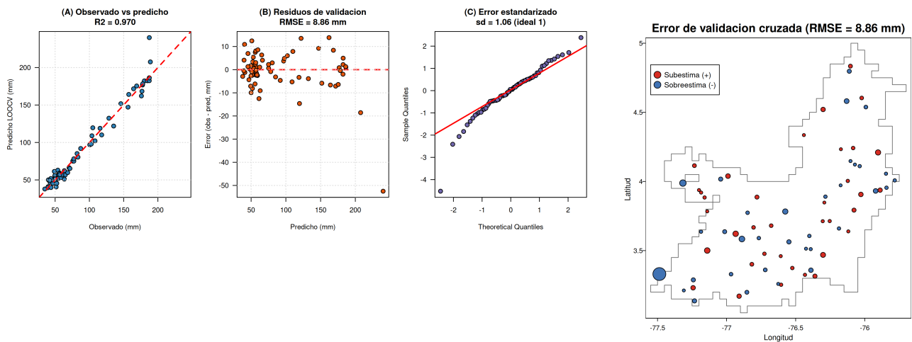
Figura 8. Izquierda: diagnóstico de la validación cruzada. Los puntos se alinean sobre la diagonal, los residuos de validación no muestran patrón contra el valor predicho, y el Q-Q del error estandarizado sigue la recta con desviación 1,06, lo que confirma que la varianza de kriging está bien calibrada y por lo tanto el mapa de incertidumbre es interpretable. Derecha: el error de validación sobre el mapa. A diferencia de los residuales de la tendencia (figura 5), aquí los colores ya no forman manchas : el kriging absorbió la estructura espacial que la regresión había dejado suelta. Es la confirmación visual de que cumplió su función.
