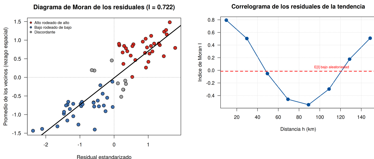
Figura 6. Izquierda: diagrama de Moran, con el residual estandarizado en el eje horizontal y el promedio de sus vecinos en el vertical; la pendiente de la recta es el índice. El predominio de rojos (alto rodeado de alto) y azules (bajo rodeado de bajo) sobre los grises discordantes es la autocorrelación positiva vista punto a punto. Derecha: correlograma, el resultado más informativo de esta sección. No es una curva que decae hasta cero y se queda ahí, sino una onda : I = +0,79 a 10 km, +0,50 a 30 km, cruza cero cerca de los 48 km, llega a -0,54 a los 89 km y vuelve a subir a +0,51 a los 149 km.
