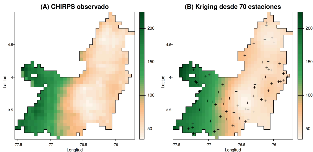
Figura 9. A la izquierda el campo CHIRPS observado y a la derecha el reconstruido por kriging universal desde solo 70 estaciones, en la misma escala de color. Se recuperan el gradiente occidente-orientado, la posición del máximo en la vertiente pacífica y las magnitudes; el mapa estimado es algo más suave, que es exactamente lo que se espera de un interpolador óptimo en media cuadrática.
