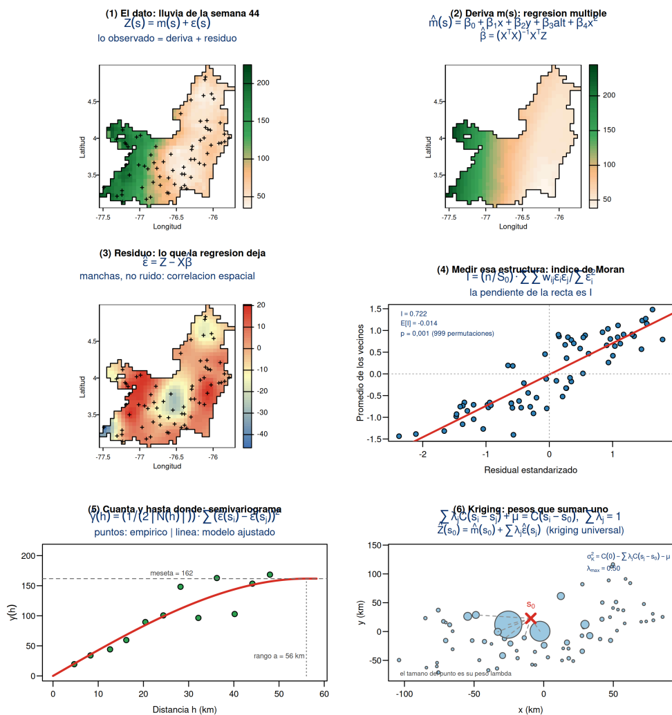
Figura 2. El método completo sobre los datos del proyecto, paso a paso. (1) El dato de partida, la lluvia de la semana 44 con las 70 estaciones sorteadas. (2) La deriva que estima la regresión múltiple: reproduce el gradiente occidente-oriente pero no los detalles. (3) El residuo, que es lo que la regresión no explicó; lo importante es que no está disperso al azar sino agrupado en manchas rojas y azules, y esa es exactamente la correlación espacial que el enunciado pide evaluar. (4) Esa estructura se mide con el índice de Moran: cada punto es una estación, el eje horizontal su residual y el vertical el promedio
